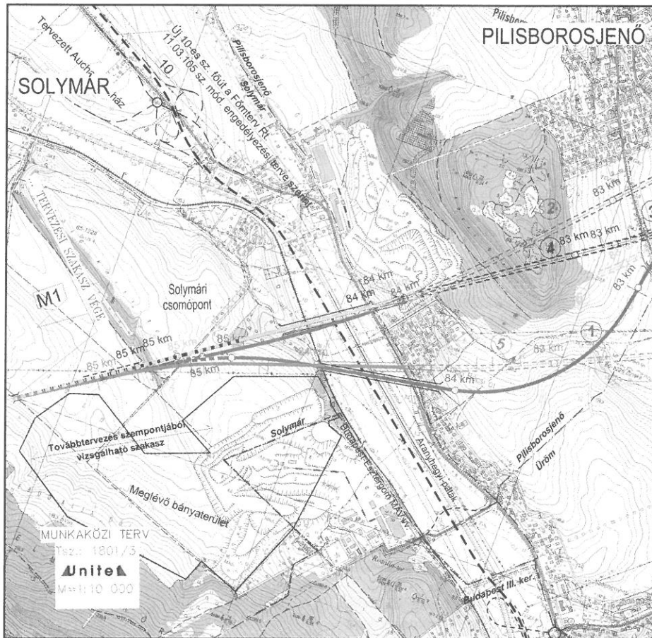
Az M0-ás és az új 10-es út kereszteződésének variációi a tanulmánytervben
